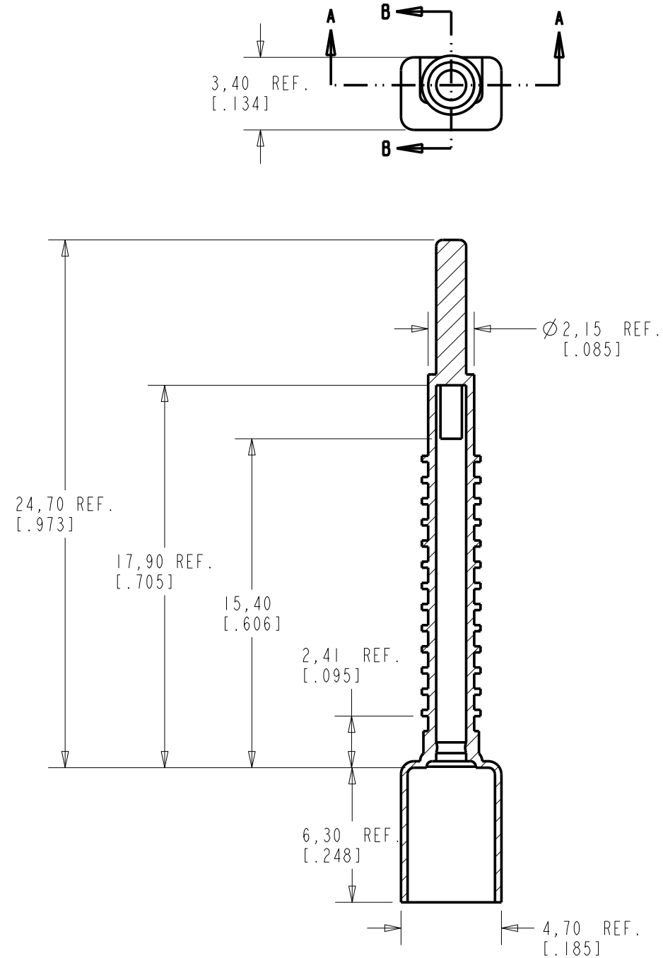
SECTION A-A
